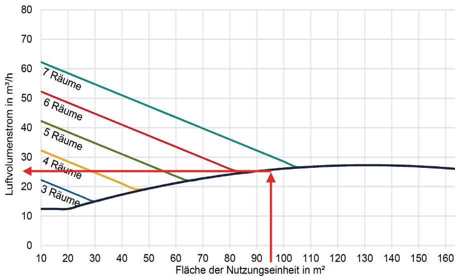
4 | Diagramm B.3: Notwendiger Volumenstrom über alle Fensterlüfter für Lüftung zum Feuchteschutz in Abhängigkeit der Fläche der Nutzungseinheit und der Anzahl der Räume:
