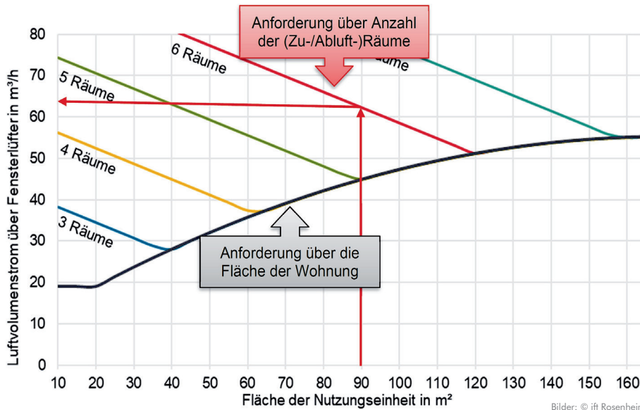
5 | Notwendiger Volumenstrom über alle Fensterlüfter für Lüftung zum Feuchteschutz in Abhängigkeit der Fläche der Nutzungseinheiten (schwarze Linie) und der Anzahl der (Zu-/Abluft-)Räume (bunte Linien) (Bild B.0 aus LU-02/2)
