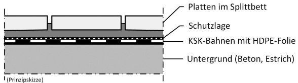
Bild 1: Abdichtung mit KSK-Bahnen mit HDPE-Trägerfolie und Platten im Splittbett auf Schutzlage. Quelle: Prof. Dr. Peter Schmidt
