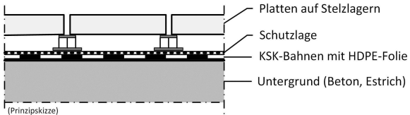
Bild 2: Abdichtung mit KSK-Bahnen mit HDPE-Trägerfolie und Platten auf Stelzlagern über einer Schutzlage. Quelle: Prof. Dr. Peter Schmidt
