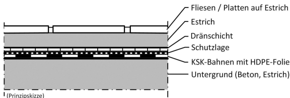
Bild 3: Abdichtung mit KSK-Bahnen mit HDPE-Trägerfolie und Fliesen oder Platten auf Estrich mit Dränschicht über einer Schutzlage. Quelle: Prof. Dr. Peter Schmidt
