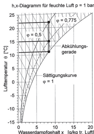
Bild 1.2: Mollier-(h, x)-Diagramm mit senkrechter Abkühlungslinie (Abkühlungsgerade) [Heinz11]
