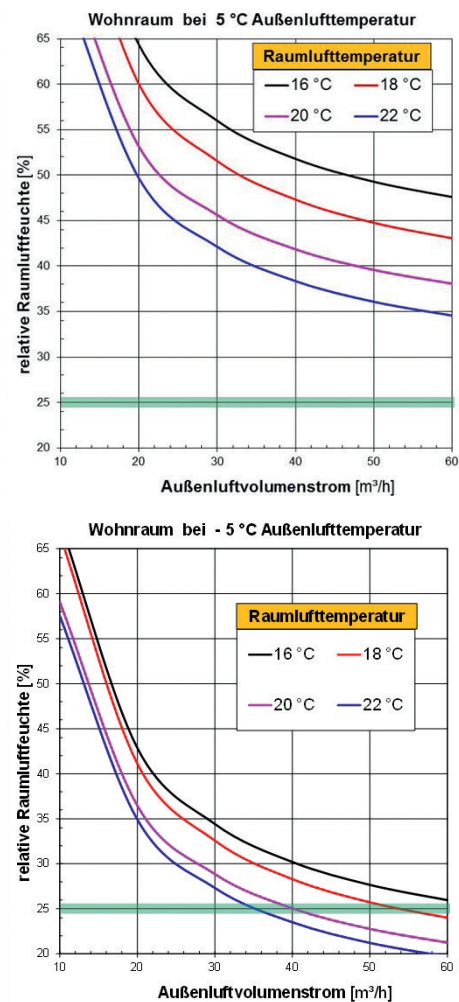
Bild 1.3: Abhängigkeit der relativen Raumlufffeuchte vom zugeführten Außenluftvolumenstrom und von der Raumlufftemperatur im Heizungsfall (Außenlufttemperatur: 5\text{ °C} und -5\text{ °C} ) (Quelle: Heinz)
